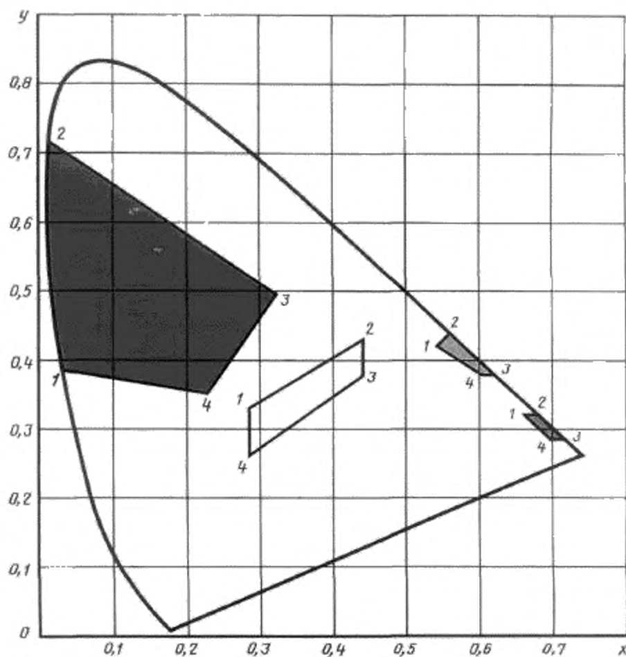
Рисунок В.1 — Границы цветовых областей выходной апертуры светофора
